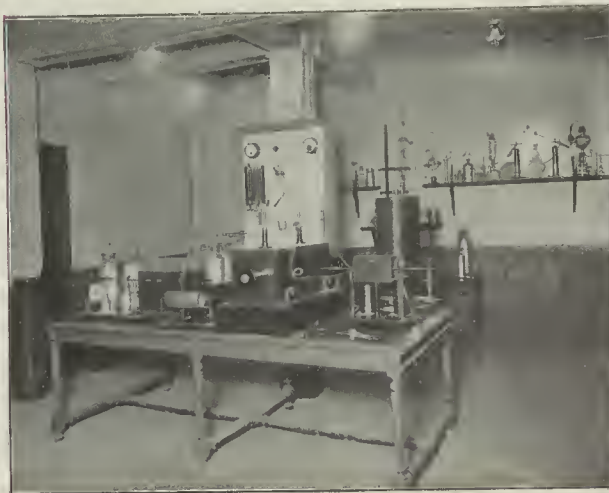
El laboratorio de experimentos en donde están instaladas las baterías eléctricas y los acumuladores
